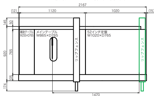
52インチ補助テーブル取付時 寸法図
